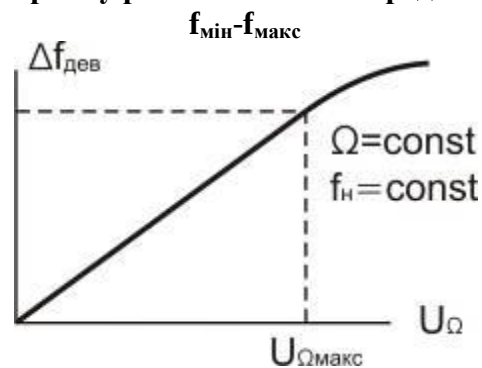
Риснок 7.20 – Характеристика сталості девіації частоти \Delta f_{\text{дев}} в будь-якій точці інтервалу робочих частот передавача f_{\text{мін}}-f_{\text{макс}}
