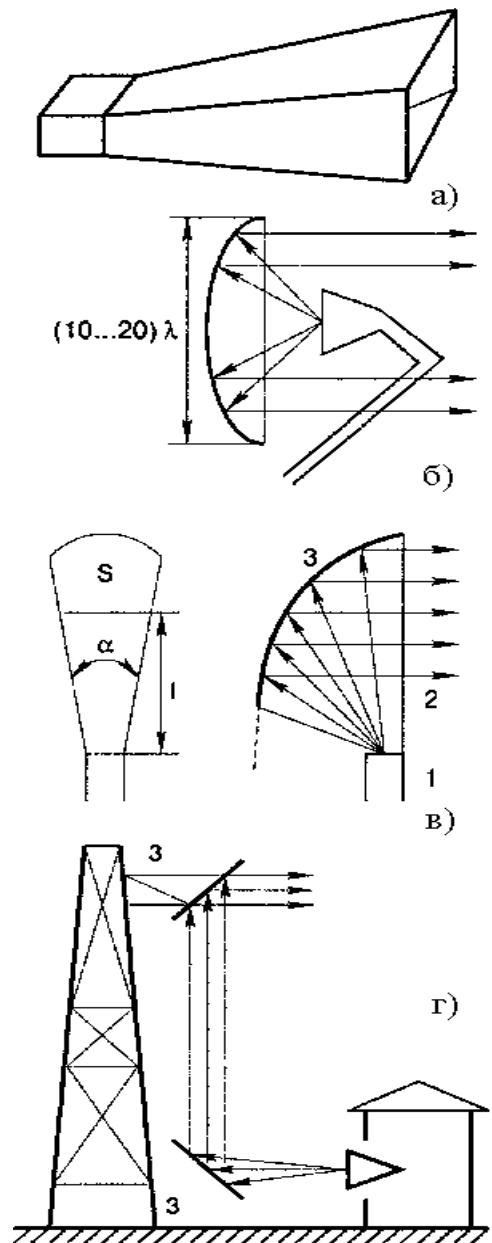
Рисунок 6.22 – Конструкції антен НВЧ:
