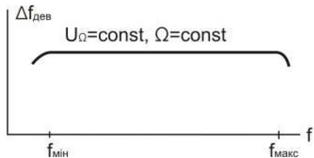
Риснок 7.20 – Характеристика сталості девіації частоти \Delta f_{\text{дев}} в будь-якій точці інтервалу робочих частот передавача f_{\text{мін}}-f_{\text{макс}}
