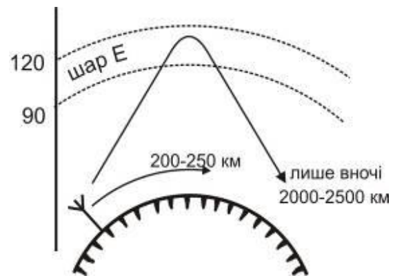
Рисунок 5.9 – Розповсюдження гектометрових хвиль
