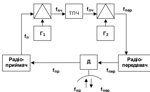
Рисунок 11.20. Структурна схема СП з двома перетвореннями та трактом проміжної частоти (ТПЧ)
