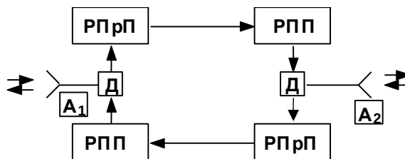
Рисунок 11.5 – Структурна схема РРЗ у режимі ретрансляції високою частотою
