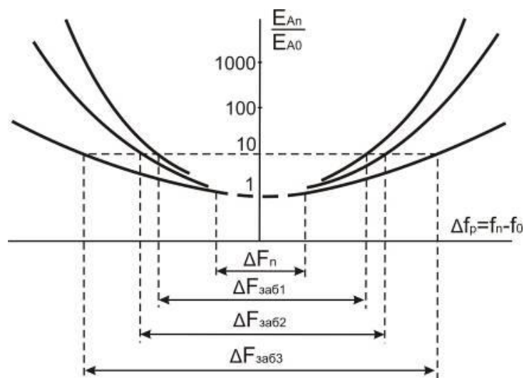
Рисунок 8.5 – Криві БСВ під впливом перешкод, що призводять до блокування радіоприймача
