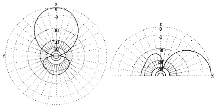
Рисунок 6.14 – Діаграма направленості чотирьохелементної антени типу "хвильовий канал"
