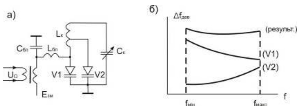
Рисунок 7.24 – Схема частотного модулятора зі змішаним включенням варикапів (а) та зміни величини діапазону частот при змішаному включенні двох варикапів у контур ЧМГ (б)
