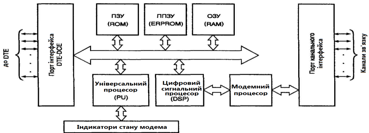
Рисунок 4.6 – Фізична структура модему
