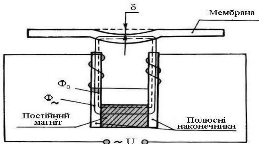
Рисунок 3.6. – Електромагнітний телефон:
