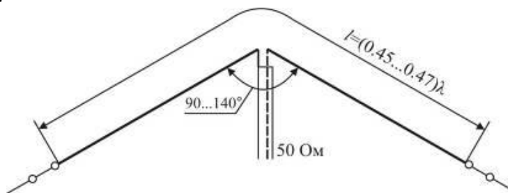
Рисунок 6.20 – Антена "перевернута V"
