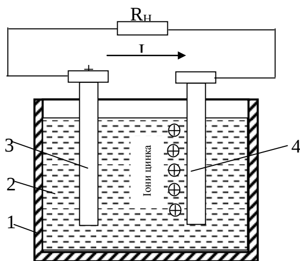
Рисунок 9.1 – Принцип дії мідно-цинкового гальванічного елемента
