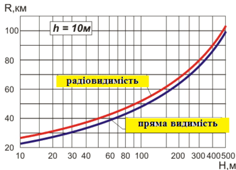
Рисунок 5.15 – Залежності оптичної та радіодальності прямої видимості від висоти підйому передаючої антени
