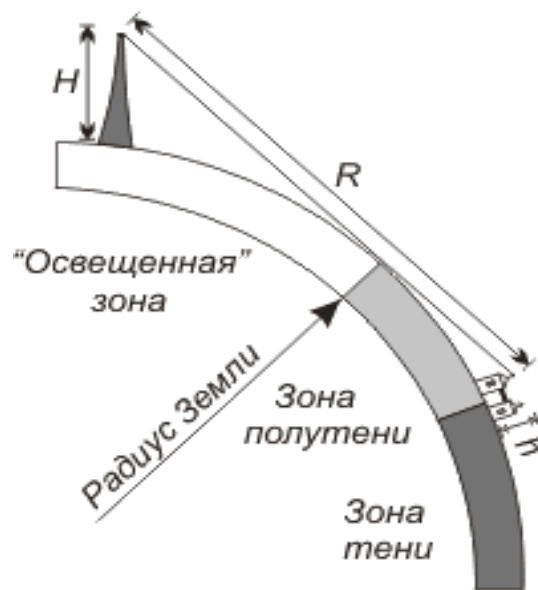
Рисунок 5.14 – Зони розповсюдження радіохвиль
