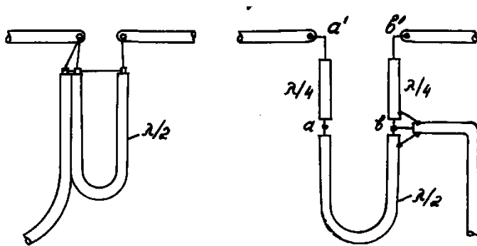
Рисунок 6.11 – Петля, що симетрує, для усунення антенного ефекту
