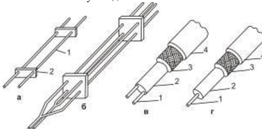
Рисунок 2.21 – Основні види ВЧ ліній передачі:
