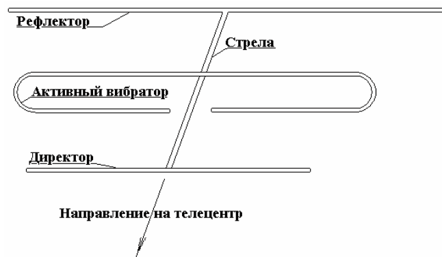
Рисунок 6.13 – Трьохелементна антена "Хвильовий канал"
