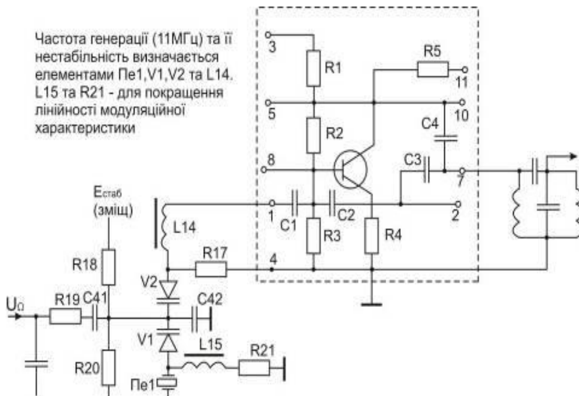
Рисунок 7.27 – Схема ЧМГ малопотужної радіостанції Р-148
