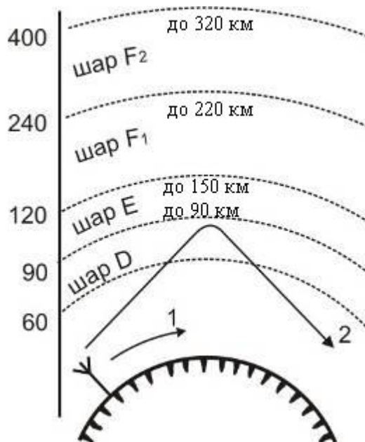
Рисунок 5.7 – Шари іоносфери:
