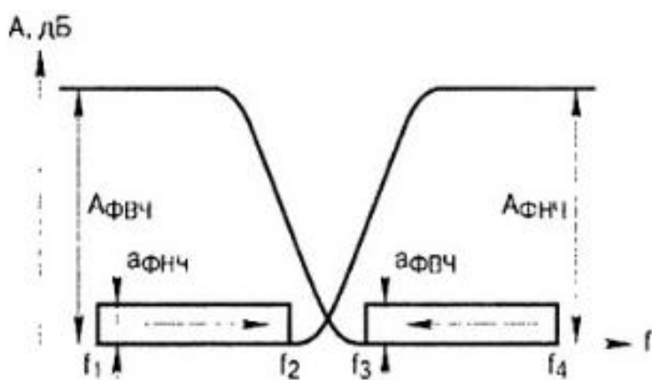
Рисунок 2.7 – Характеристики послаблення фільтрів верхніх і нижніх частот:
