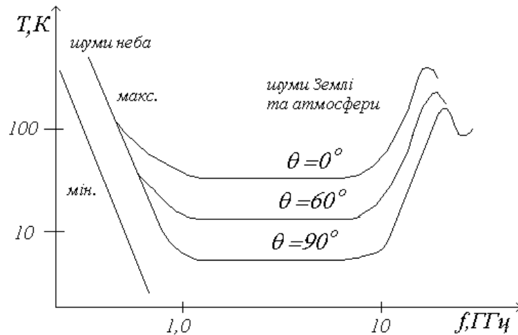
Рисунок 8.2 – Якісний характер частотних залежностей джерел зовнішніх завад Λ
