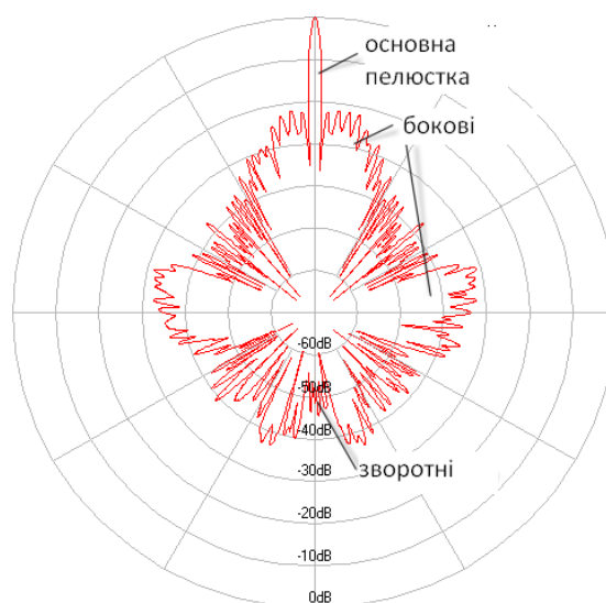
Рисунок 6.6 – Площинна ДНА
